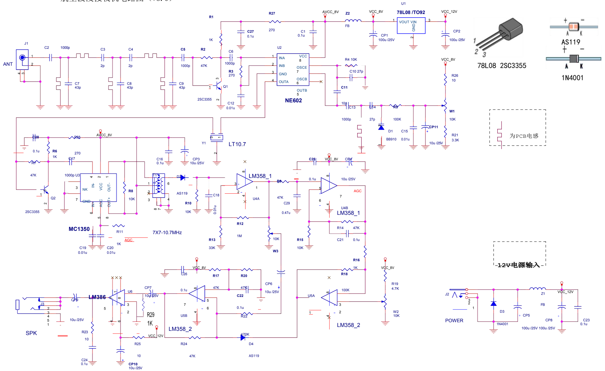
航空波段接收机电路图 (V3.0)
